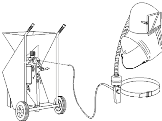
Branchement direct sur une sableuse ARENA
